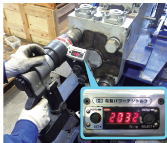
電動パワーレンチによるトルク管理
