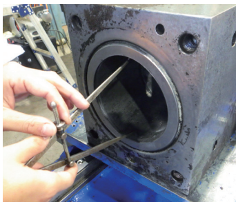
充実した測定器具による消耗部品の測定
